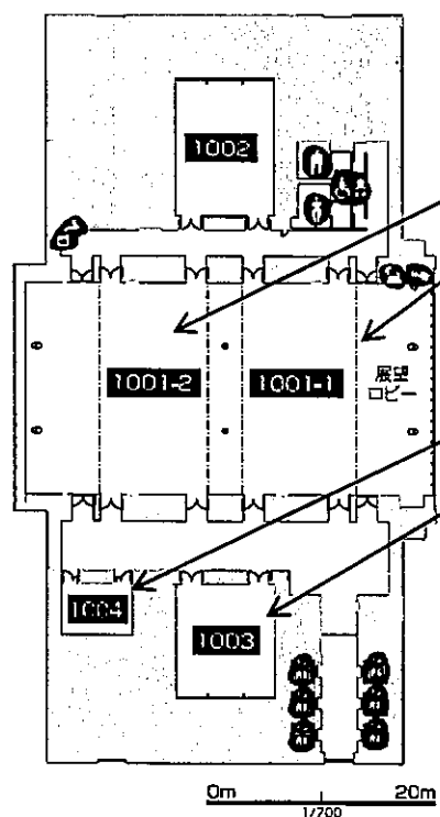
10F全体配置図
